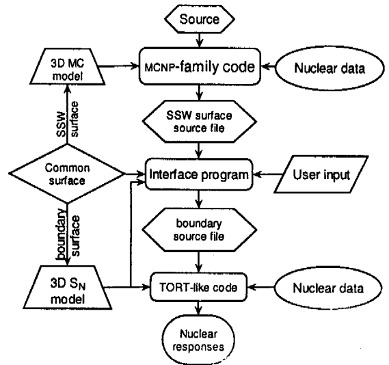
图 1 三维耦合屏蔽计算程序系统
