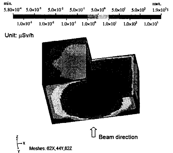
图 4 IFMIF 维修大厅剂量分布
