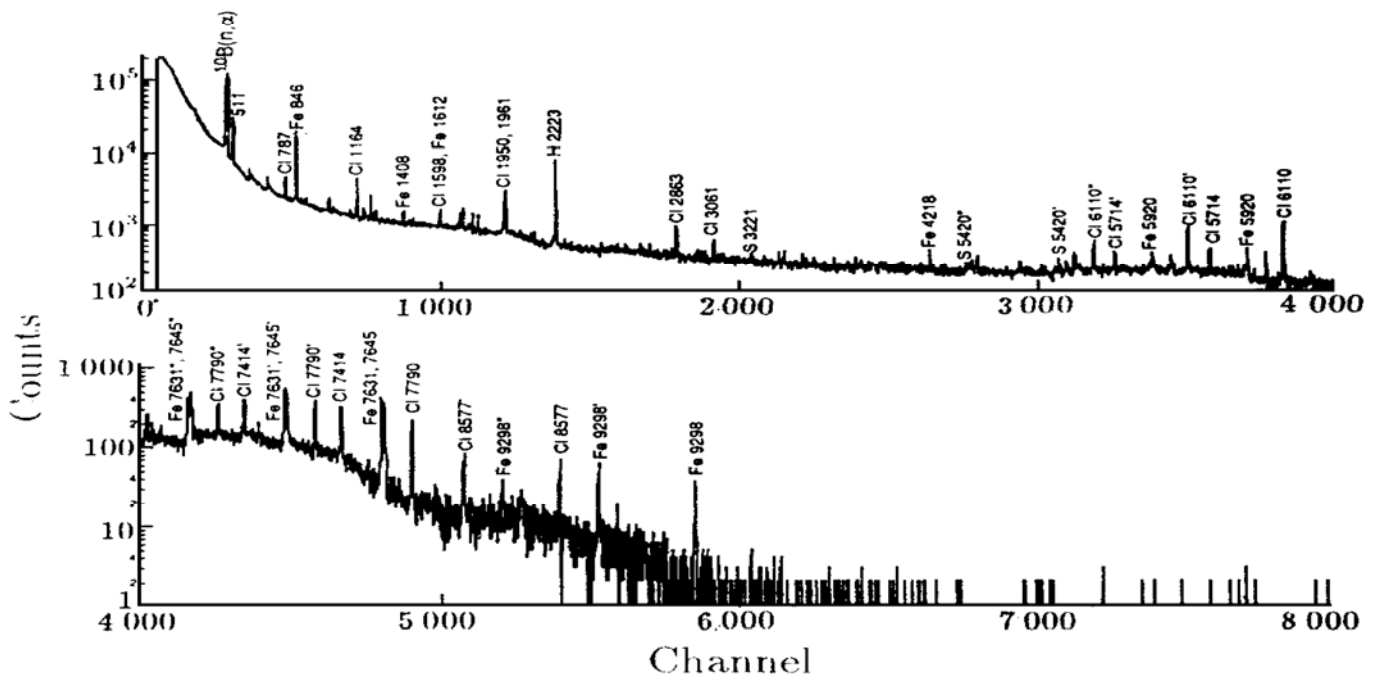
图1 化学毒剂 HD 的中子诱发 \gamma 谱 [2]
