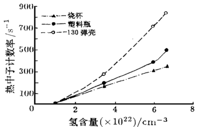
图 2 热中子计数率与氢含量的刻度曲线
