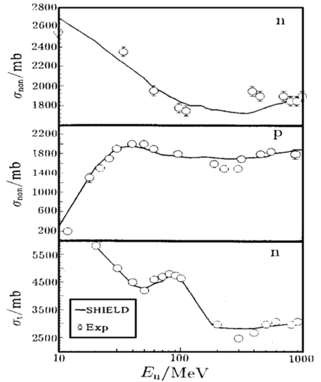
图 1 SHIELD 计算 n(p) + {}^{208}\text{Pb} 的非弹和总截面
