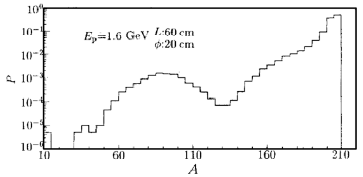
图5 SHIELD 计算1.6 GeV 质子入射 nat Pb 厚靶碎片分布
