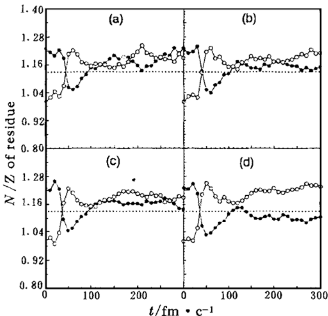
图1 ^{40}\text{Ca} + ^{58}\text{Fe} 反应系统对心碰撞时体系左边 ( z < 0 , \circ ) 和右边 ( z > 0 , \bullet ) N/Z 的时间演化
