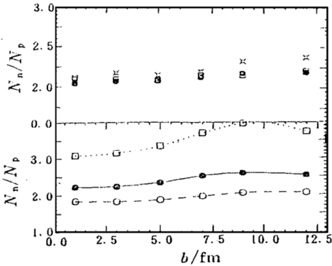
图2 轰击能量为40 MeV/u ^{132}\text{Sn} + ^{132}\text{Sn} 反应系统中总的非平衡中子和质子比与碰撞参数的关系
