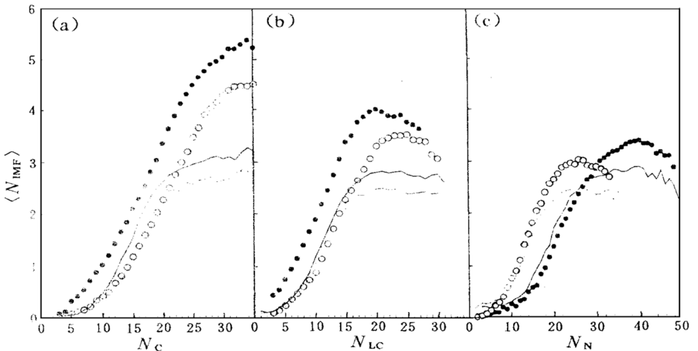
图4 40 MeV/u ^{112}\text{Sn} + ^{112}\text{Sn} 和 ^{124}\text{Sn} + ^{124}\text{Sn} 反应系统中 \langle N_{\text{IMF}} \rangle 随 N_C (a)、 N_{\text{LC}} (b) 以及 N_N (c) 的变化关系
