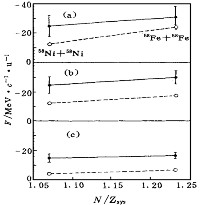
图3 轰击能量为55 MeV/u ^{58}\text{Fe} + ^{58}\text{Fe} 和 ^{58}\text{Ni} + ^{58}\text{Ni} 反应系统中, 3种碎片的流参数和系统的 N/Z 关系 \bullet 计算值, \circ 实验值, (a) Z = 3 , (b) Z = 2 , (c) Z = 1 .
