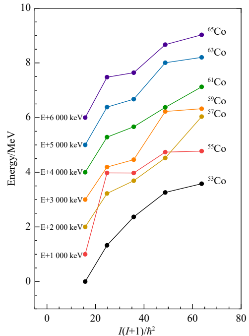
图 2 奇 A 核 Co 同位素链负宇称晕态能量 [48] 随 I(I+1) 的变化图 (在线彩图)
