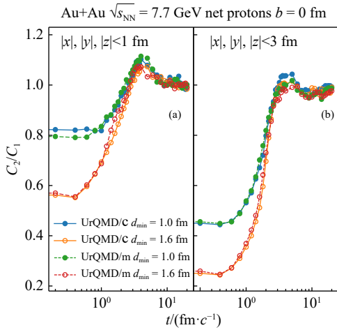
图 4 在碰撞参数 b = 0 fm 时，坐标空间中心区域净质子数 C_2/C_1 随时间的演化 (在线彩图)
