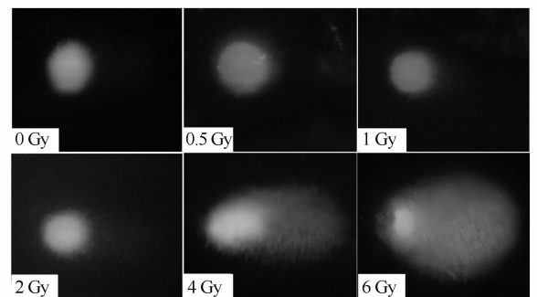
图 1 不同剂量 ^{12}\text{C}^{6+} 离子束 ( \text{LET} = 30 \text{ keV}/\mu\text{m} ) 辐照人类肝 L02 细胞荧光显微镜下的彗星图像
