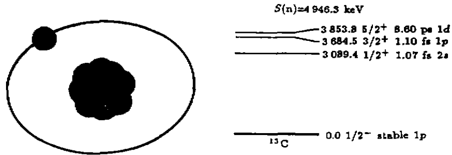
图 8 ^{13}\text{C} 1/2^- 激发态是质子晕态的示意图
