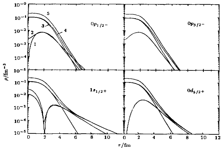
图 9 ^{13}\text{C} 基态和三个激发态实验和理论计算的密度分布
