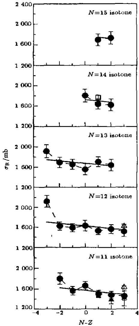
图 5 由中能 36 Ar 轰击 Be 靶产生的一系列缺中子核素的在碳靶上的反应总截面实验结果 — 是以 r_0 A^{1/3} 计算的反应总截面.
