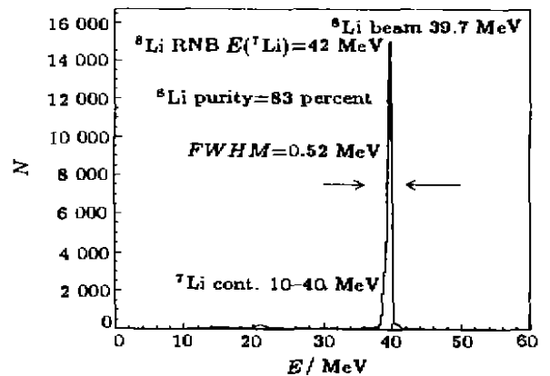
图 7 北京串列加速器实验室的低能放射性束线 GIRAFFE 最近得到的高纯度 8 Li 放射性束的能谱
