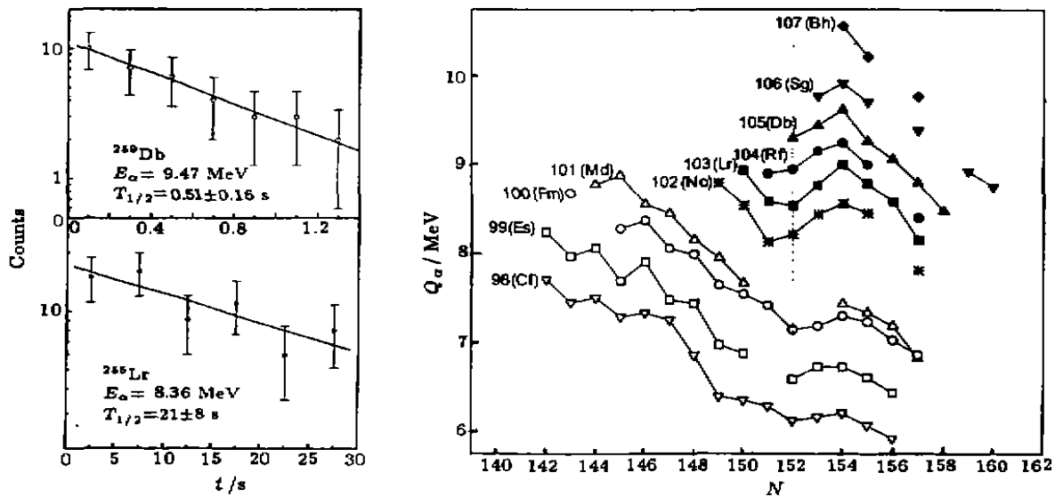
图 2 ^{259}\text{Db} 及其子体 ^{255}\text{Lr} 的半衰期测量曲线及部分重元素的 Q_\alpha 随核内中子数、质子数变化的曲线
