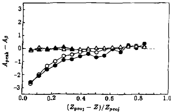
图 4 ^{36}\text{Ar} ( \blacktriangle ), ^{40}\text{Ar} ( \bullet )束轰击 Be 靶得到的碎裂反应同位素分布(原子序数为 Z 的产物)的峰位和反应剧烈程度 (Z_{\text{proj}} - Z)/Z_{\text{proj}} 的关系曲线 \triangle 和 \circ 是扩展统计碎模型的计算结果.
