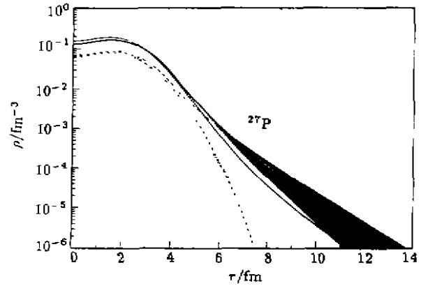
图 6 假定核子分布是 HO 型加指数尾巴、Glauber 模型拟合实验反应总截面提取的 27 P 的核物质密度分布 阴影区表示实验反应总截面误差导致的提取出的核物质密度分布的误差, 粗的——是 RMF 计算的核物质密度分布, 细的——和——是二种参数下 RMF 算出的质子和中子密度分布, 显示 27 P 可能是质子晕核.
