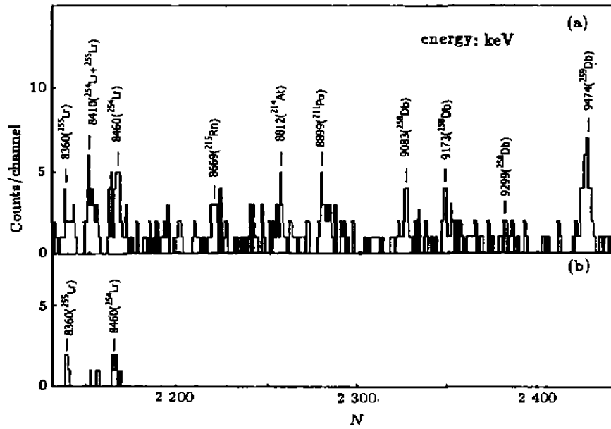
图 1 120 MeV ^{22}\text{Ne} + ^{241}\text{Am} 反应中测到的 105 号元素的同位素 ^{259}\text{Db} 的 \alpha 衰变能谱 (a)探测器面对产物样品，(b)产物样品移去后。
